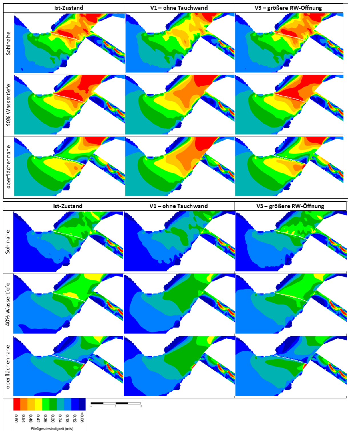
Abbildung 68: Strömungsmodellierung (3 Varianten – je 3 Wassertiefen) des Bereichs um die Tauchwand für einen Thaya-Abfluss von 3 m³/s (oben) und 1,8 m³/s (unten).
