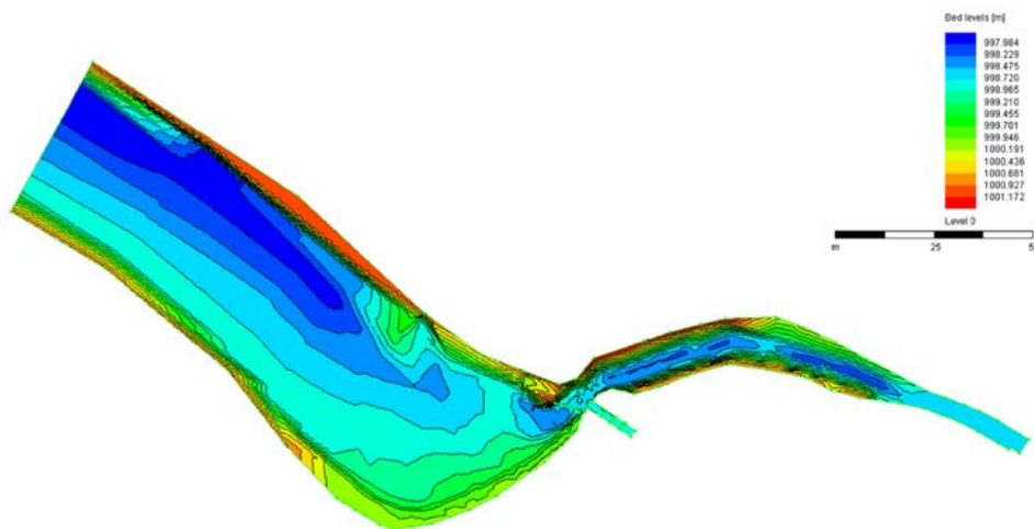
Abbildung 66: Digitales Geländemodell der modellierten Strecke (unterer Staubereich, obere FAH und Triebwasserkanal). Höhenangaben in m beziehen sich auf lokales System (relative Werte).
