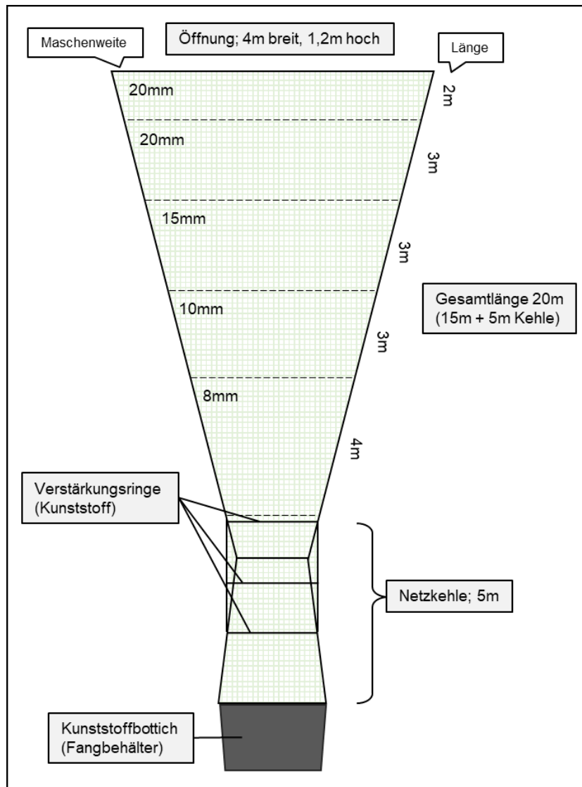
Abbildung 23: Skizze des Fanghamens und verwendete Maschenweiten. Länge des Hamens: 15m + 5m Steert (Netzreuse). In den Steert waren eine Kehle sowie ein Reißverschluss eingearbeitet.
