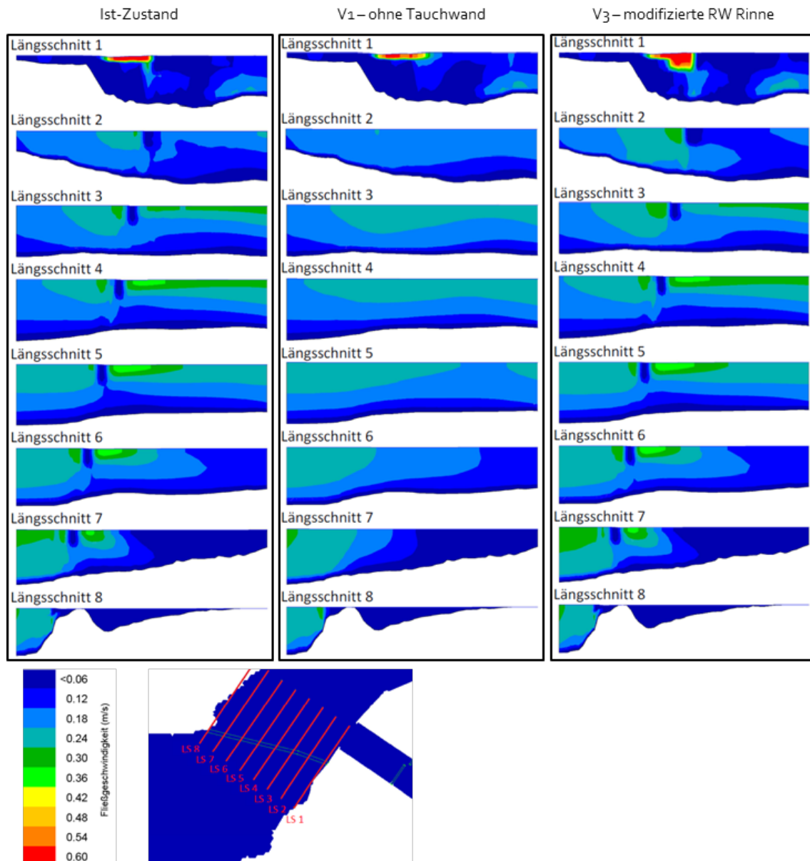
Abbildung 69: Darstellung der Strömungsgeschwindigkeiten normal zu den Strömungsprofilen bei einem Abfluss von 3 m³/s. rechts: Lage der einzelnen Profile im Bereich der Tauchwand bzw. FAH und Wehrdotation.
